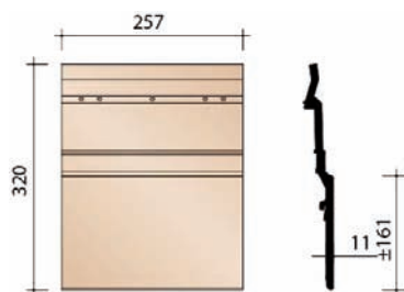
EINDSTUK FAÇATILE
